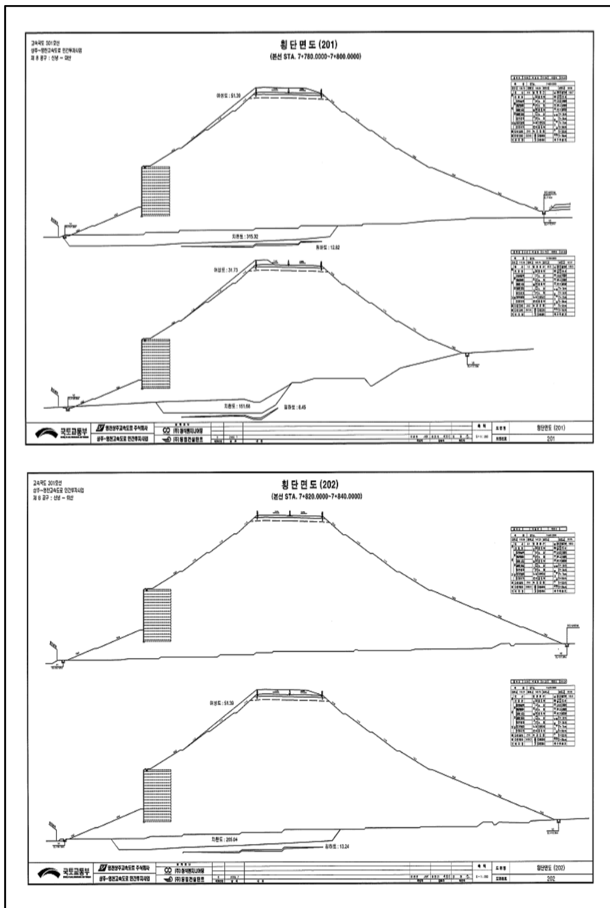
【그림 79.5】 단면도
