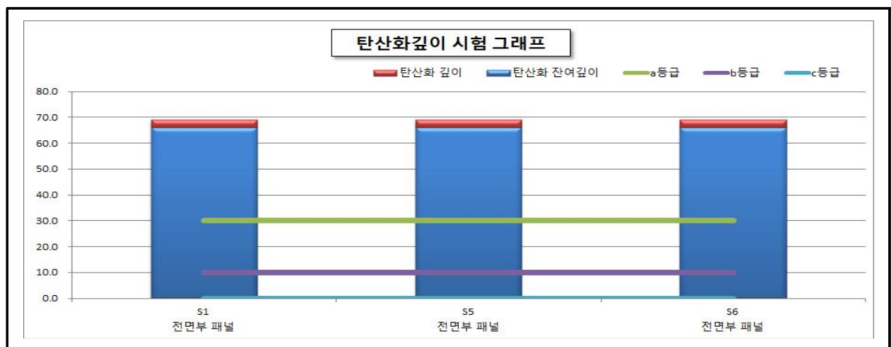
【그림 79.8】 탄산화 깊이 측정결과
