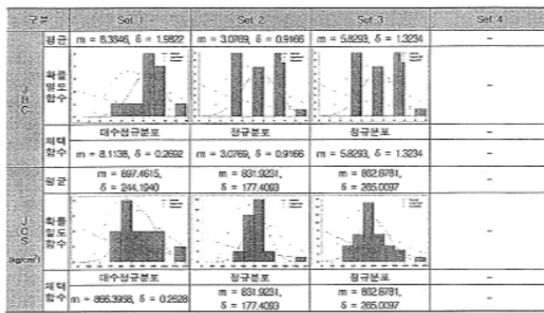
▷ Scanline L-5의 불연속면 특성
