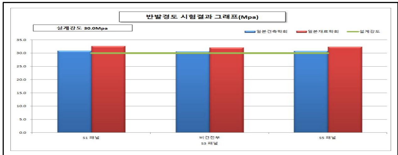
【그림 79.7】 반발경도시험 측정결과
