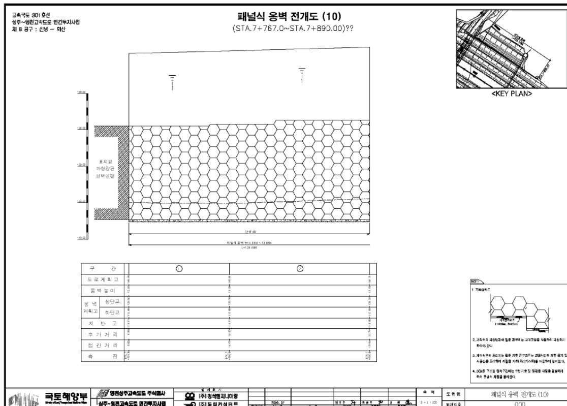
【그림 79.4】 전개도
