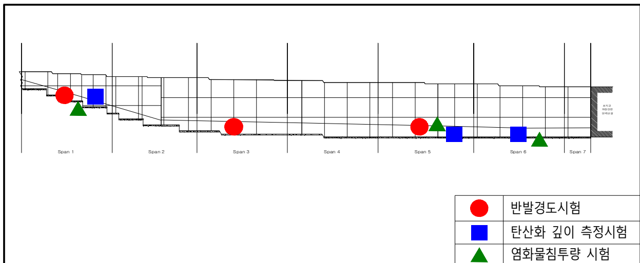
【그림 79.6】 콘크리트 재료시험 조사 위치도
