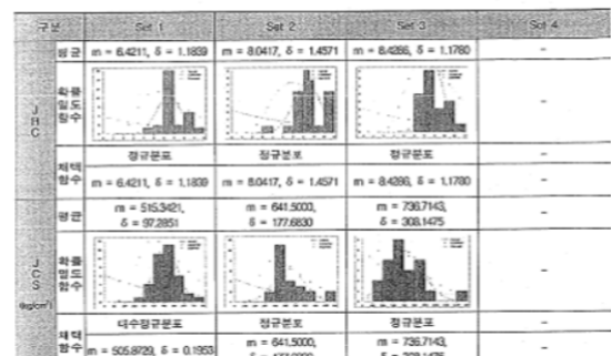
▷ Scanline SCB-5의 불연속면 종합
