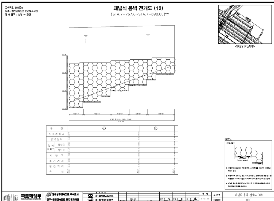
【그림 13.4】 전개도(계속)
